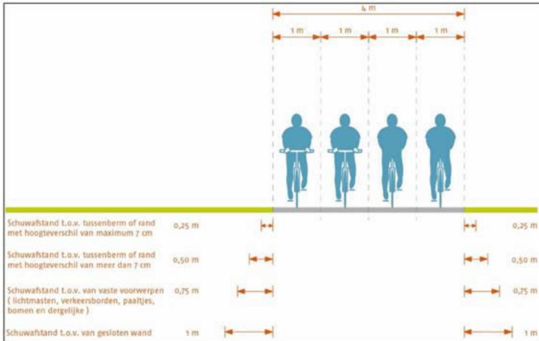
Figuur 2.3: Maatgevend gebruik fietssnelweg (2+2 fietsers)
